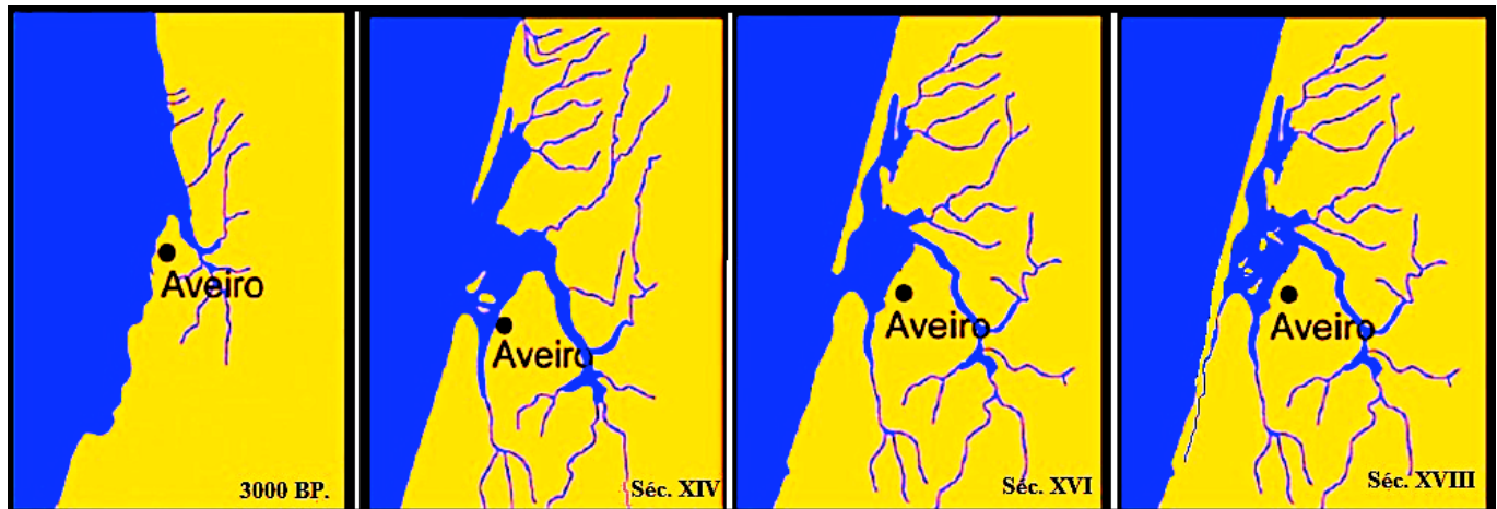
Figura 3. Evolução Geomorfológica da laguna de Aveiro (Adaptado BASTOS et al. , 2015).
